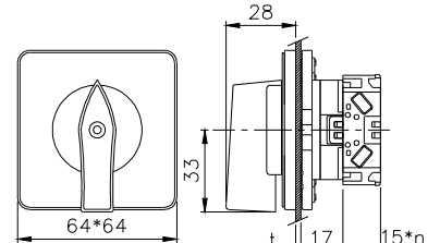
t(板厚)=8max n=p數
