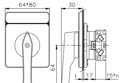
t(板厚)=8max n=p數
