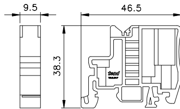
TBU2.5N-F TBU-2.5N擋片 (適用於2.5N~16N)
