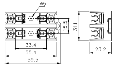
TFBR-102 (可用於TBR-N軌道)
