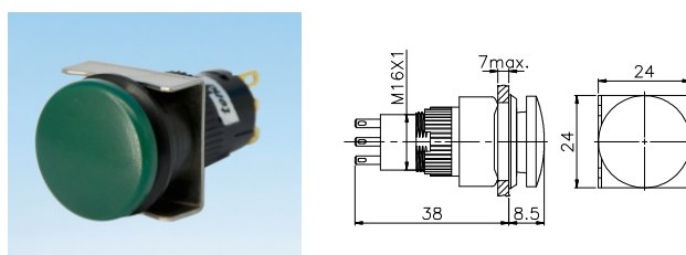
TTR16-MMBR
