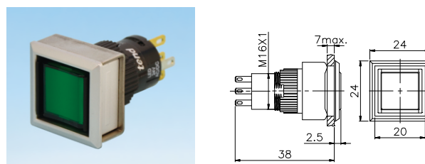
TTR16-ABFS/MBFS
