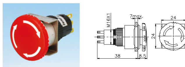
TTR16-BKLFR
