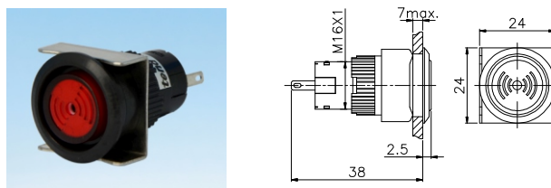
TTR16-BILBS
