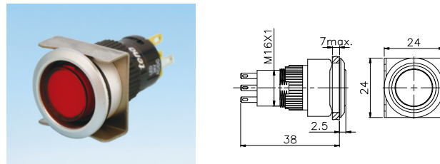
TTR16-ABFS/MBFS
