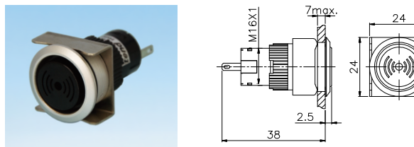
TTR16-BIFS
