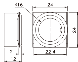
端子套 TT16-TC
